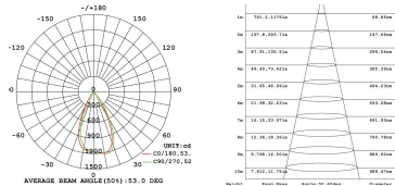
Beam angle : 50°
