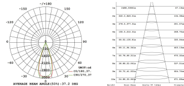
Beam angle : 36°
